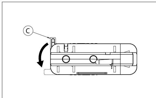
Fig. 4 Rotazione camma Pic. 4 Cam rotation
